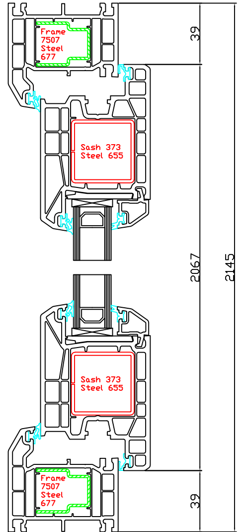
SCHNITT A-A
