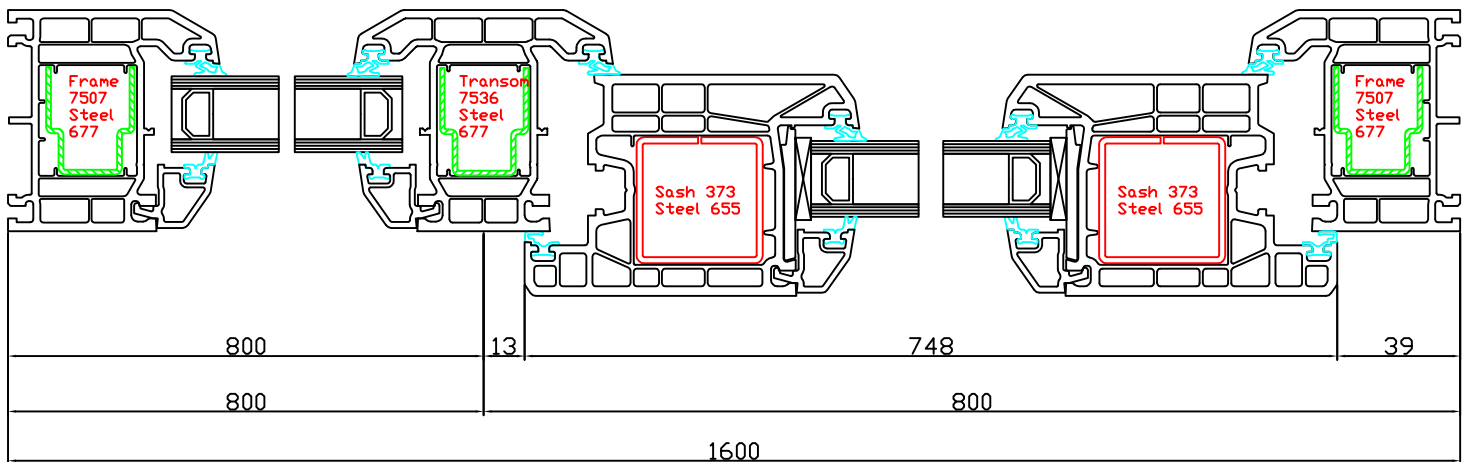
SCHNITT B-B
